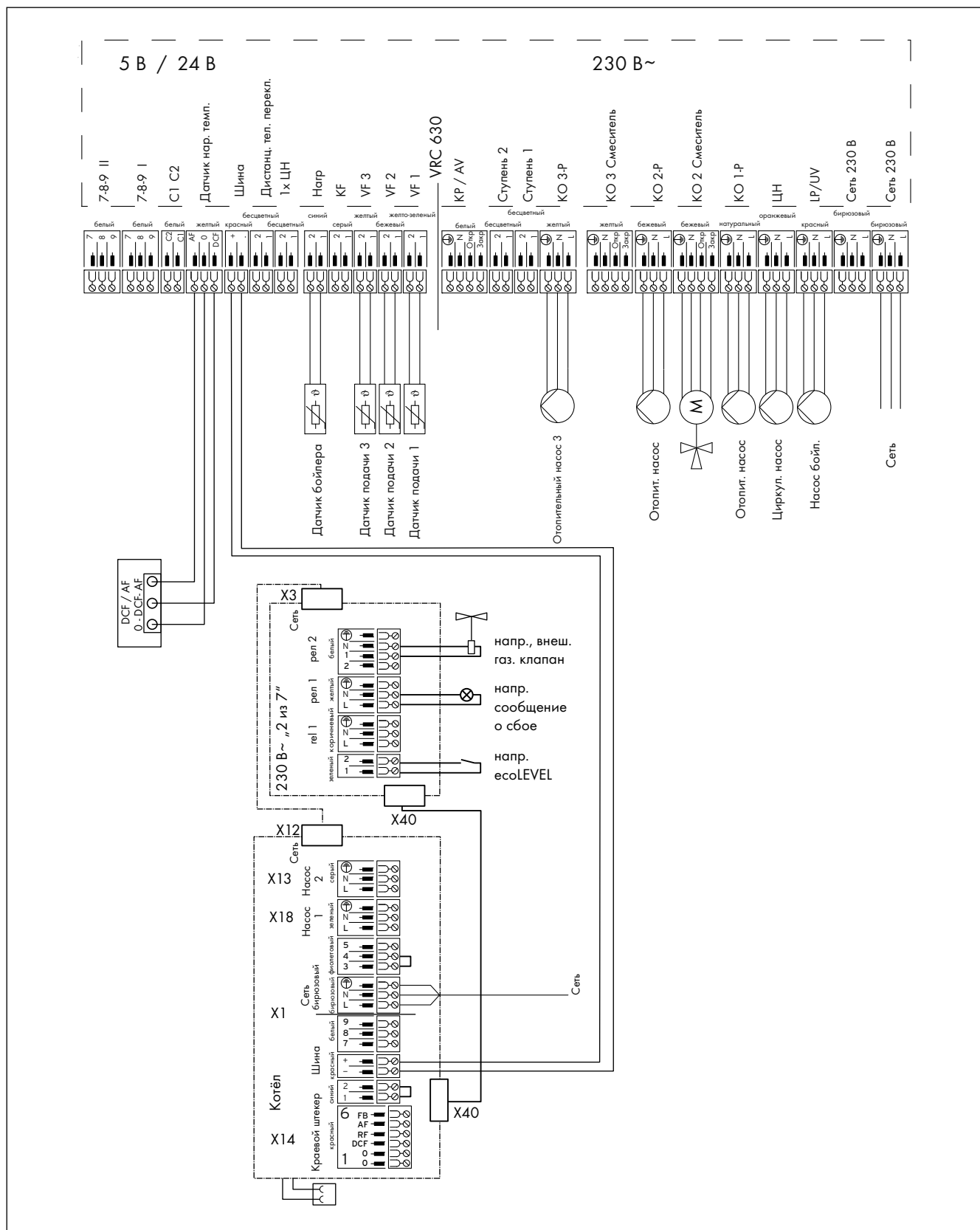
Рис. 5.15 Подключение регулятора VRS 620 или VRC 630
