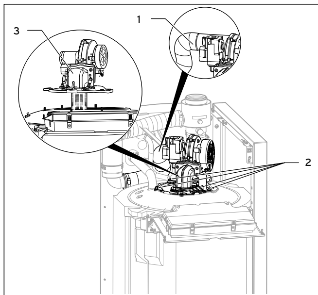
Рис. 8.2 Установка горелки
